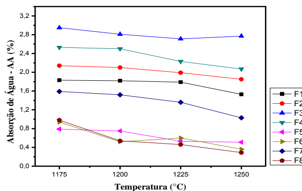
Figura 2. Ensaio de absorção de água (%) dos corpos-de-prova.
