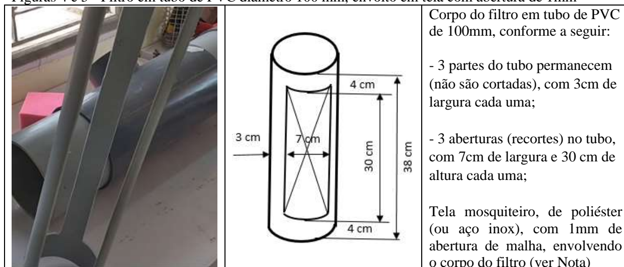
Figuras 4 e 5 - Filtro em tubo de PVC diâmetro 100 mm, envolto em tela com abertura de 1 mm
